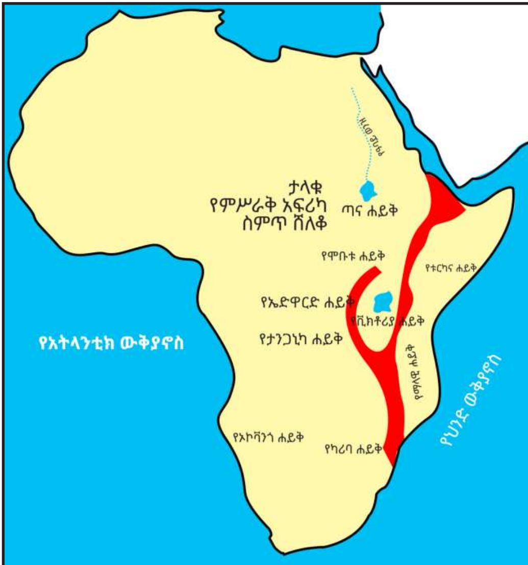
ምስል 1.8 የምሥራቅ አፍሪካ ታዋቂ ቦታዎች (ሥምጥ ሸለቆ፣ ወንዞችና ሐይቆች)
