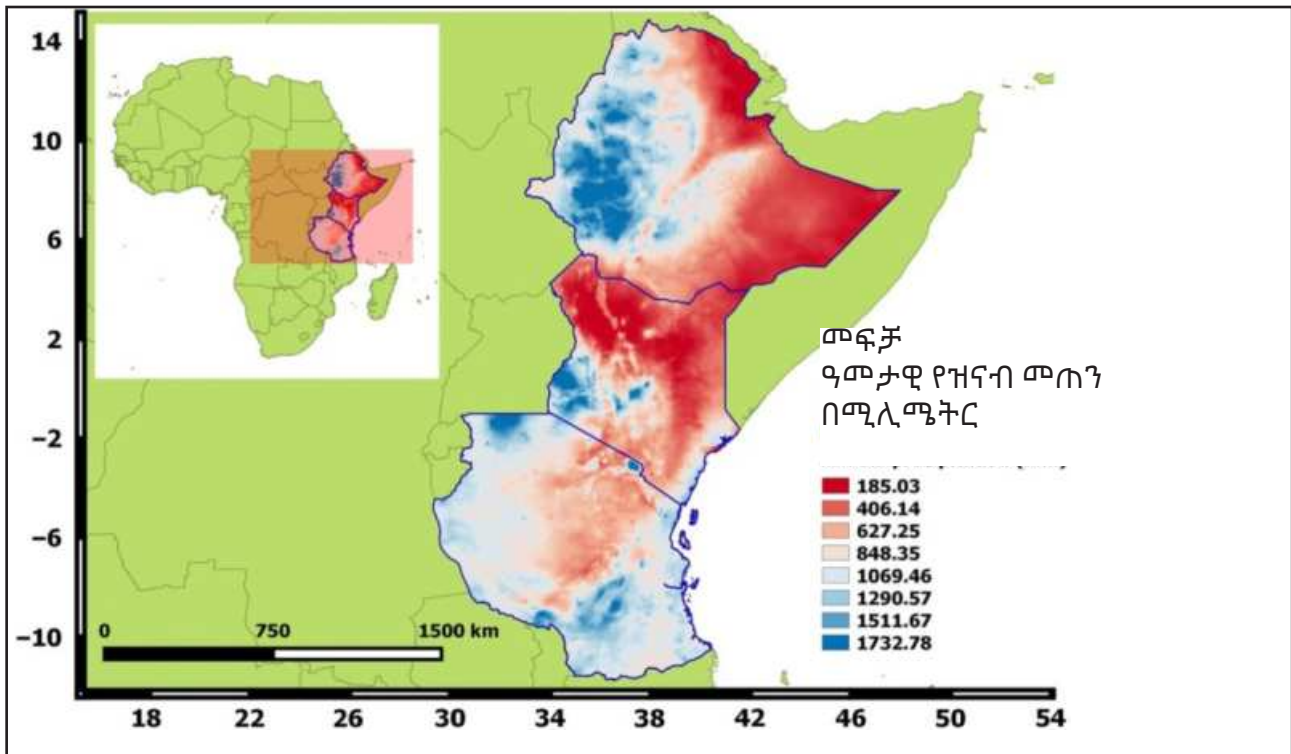
ምስል 3.2 የምሥራቅ አፍሪካ አመታዊ የዝናብ መጠን
