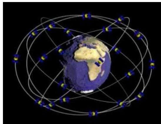
ምስል 1.15 (ለ) 2 የጂ.ፒ.ኤስ ሳተላይቶች መሬትን ሲዘሩ
