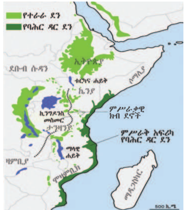
ምስል 3.8 የምሥራቅ አፍሪካ የደን ሽፋ
