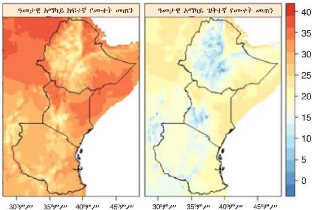
ምስል 3.1 የምሥራቅ አፍሪካ ሀገራት ወቅታዊ የሙቀት ሥርጭት ስርጭት
