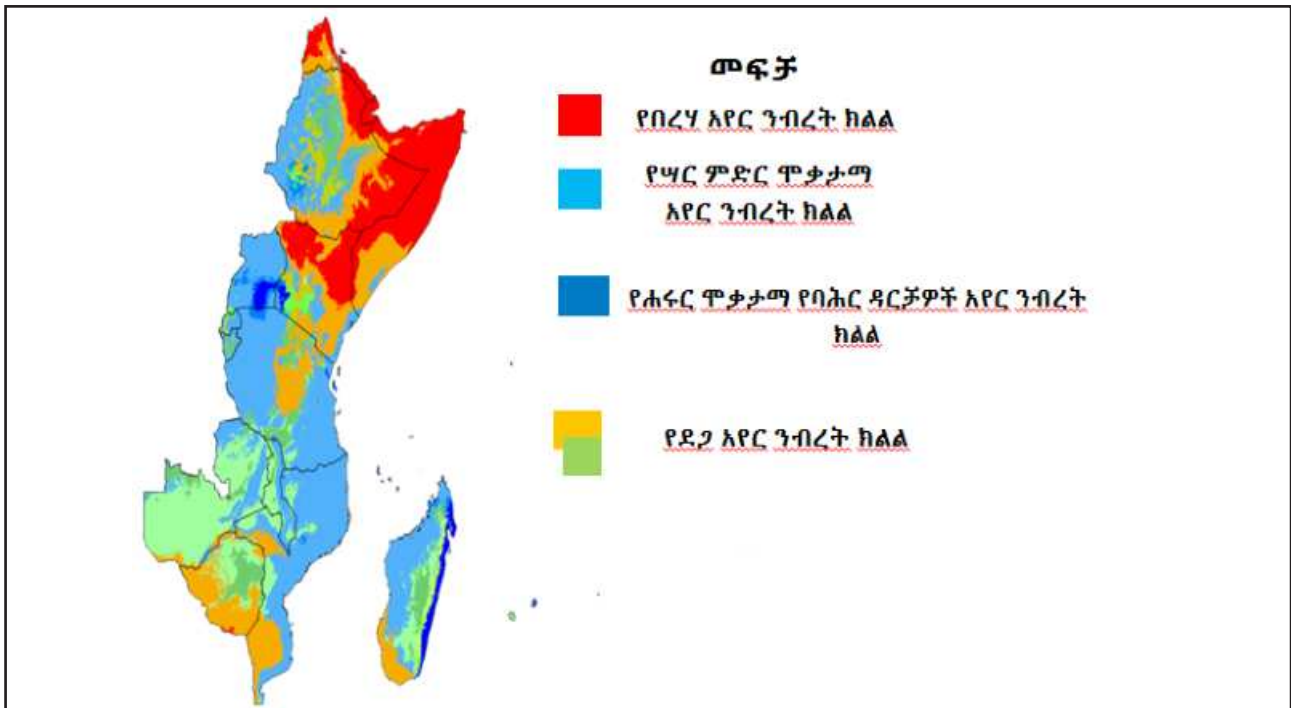
ምስል 3.2 የምሥራቅ አፍሪካ የአየር ንብረት ክልሎች
